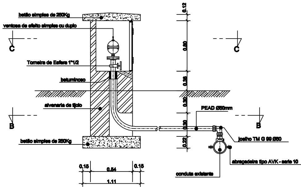
CORTE A-A
